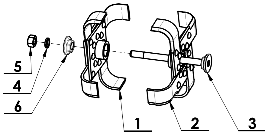
Rotační plečka APL-348 (15cm )
