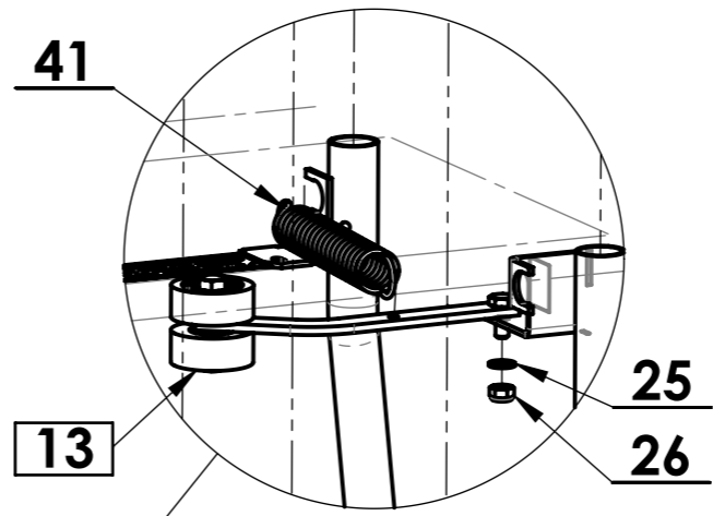
DETAIL A MĚŘITKO 1 : 5
