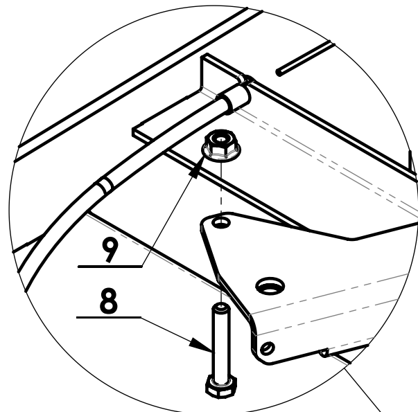
DETAIL A MÉRITKO 1:2
